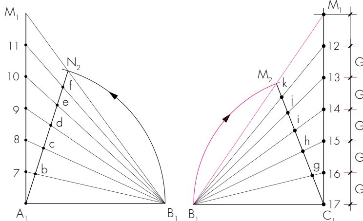
A. BALANCEMENT DES 6 MARCHES SITUÉES AVANT LE POINT M
