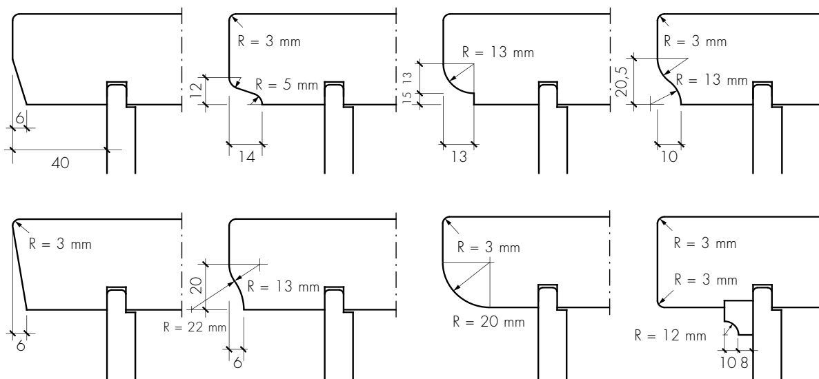
Fig. 26 Nez de marche profilés.
