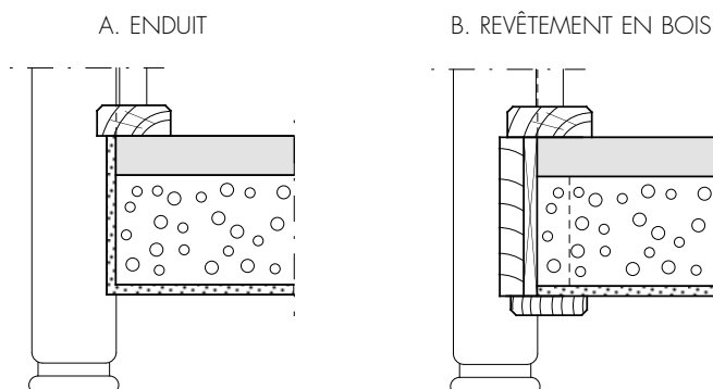
Fig. 67 Finition des rives de la trémie.
