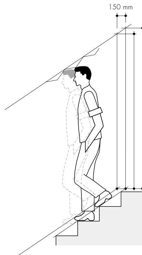
Fig. 33 Descente aisée d'un escalier.
