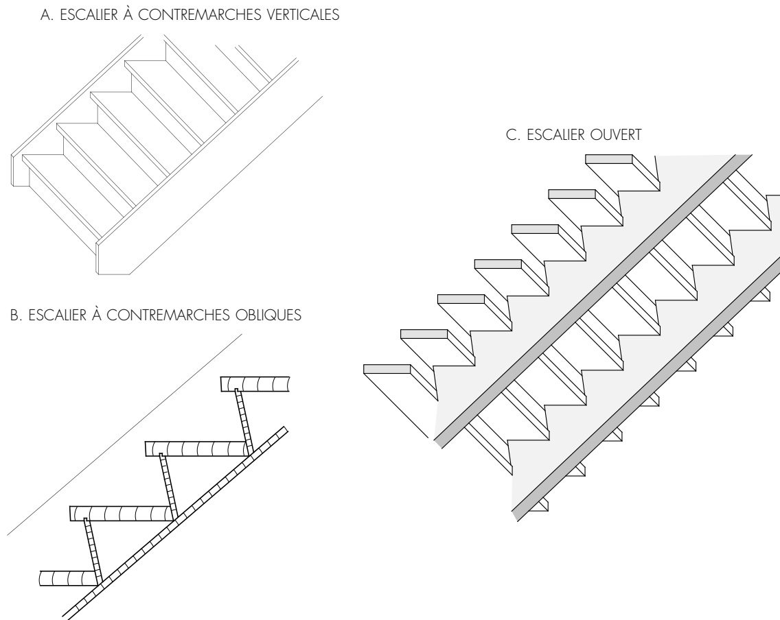
Fig. 12 Escaliers ouverts ou fermés (avec ou sans contremarches).
